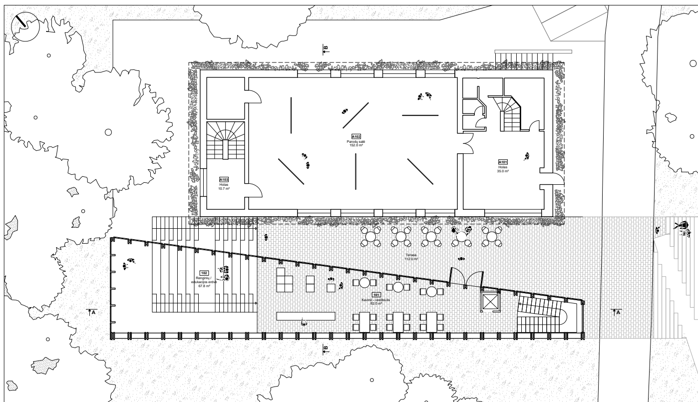
1 aukšto planas
